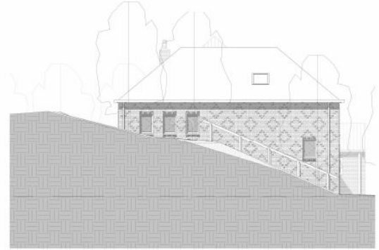
Noordoost gevel
